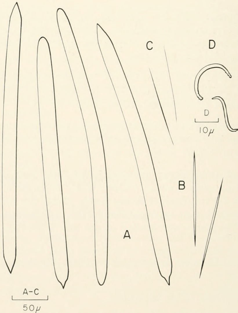
FIGURE 3. Spicules of Neofibularia nolitangere oxecta subsp. nov. A. Oxeas, style, strongyle. B. Microxeas. C. Raphides. D. Sigmas. YPM No. 7604. Holotype.
