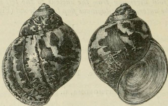
Saulea vitrea .
