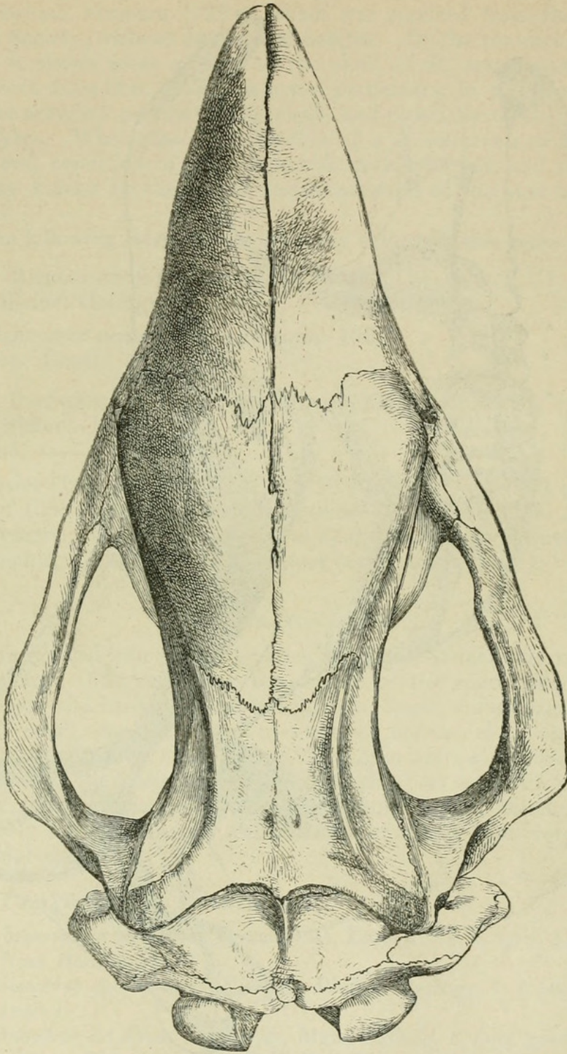
Rhinoceros stenocephalus.
