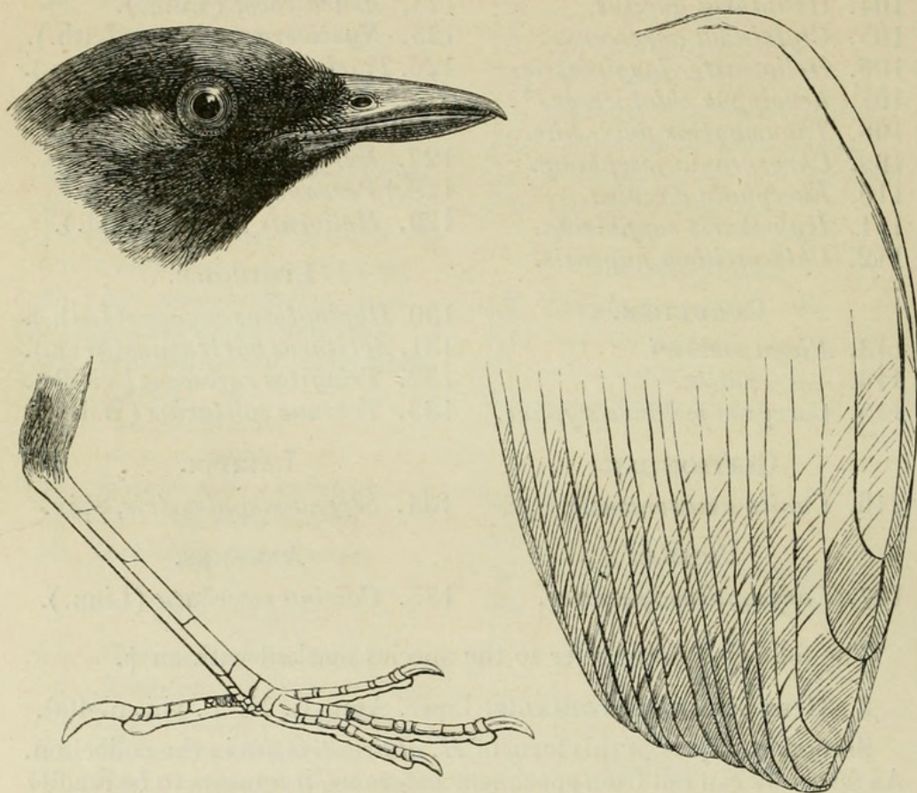
Percnostola fortis.
