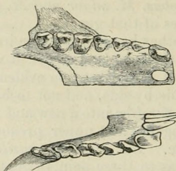
Lepilemur mustelinus .
