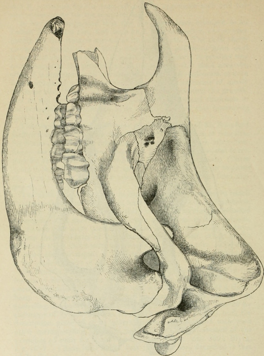
Rhinoceros stenocephalus.
