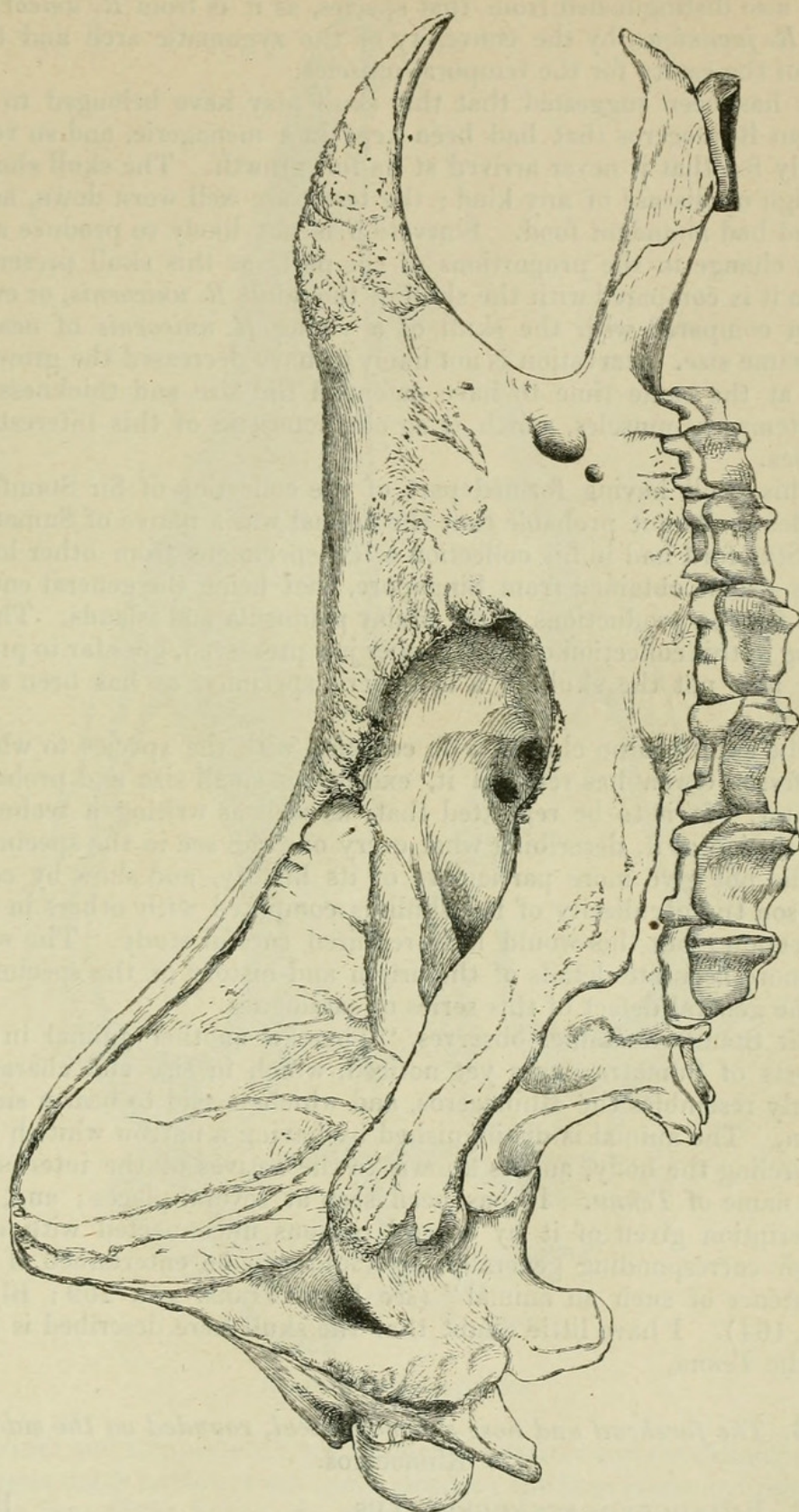
Rhinoceros floweri.
