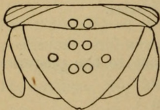
FIG. 13.— SPHÆROMA OCTONCUM . \times 13\frac{1}{2} . ABDOMEN.
