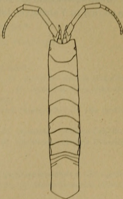
FIG. 20.—IDOTEA RECTILINEATA LOCKINGTON. \times 2 .
