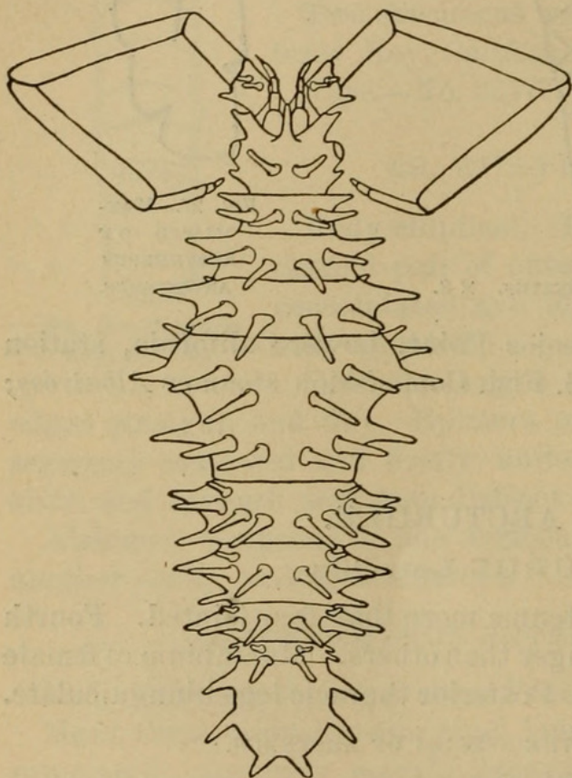
FIG. 28.—ARCTURUS INTERMEDIUS. X 10.
