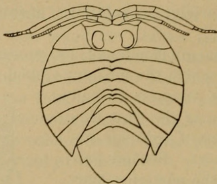
FIG. 19.—SEROLIS CARINATA LOCKINGTON. \times 8 .
