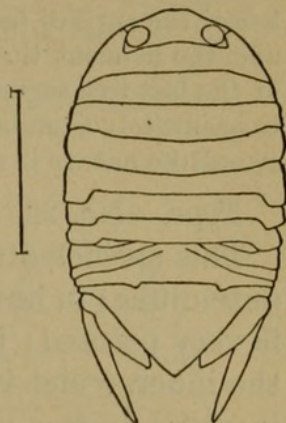
FIG. 14.—TECTICEPS ALASCENSIS RICHARDSON. \times 2\frac{1}{2} .
