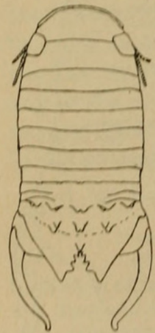
FIG. 17. — CILICÆA CAUDATA GILLIANA . × 8.
