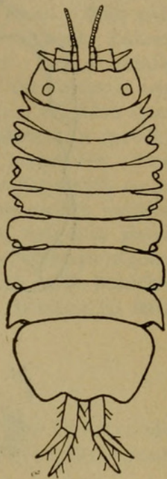
FIG. 30.— IANTHE EROS-TRATA . \times 13\frac{1}{2} .
