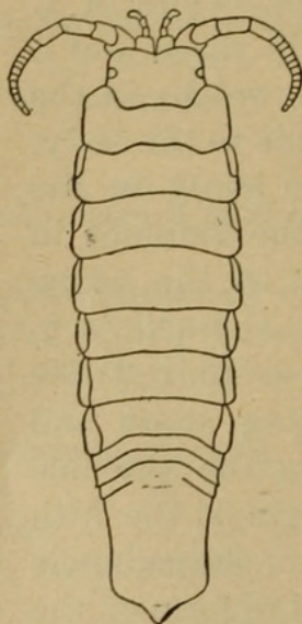
FIG. 21.—IDOTEA OCHOTENSIS BRANDT. × 2.
