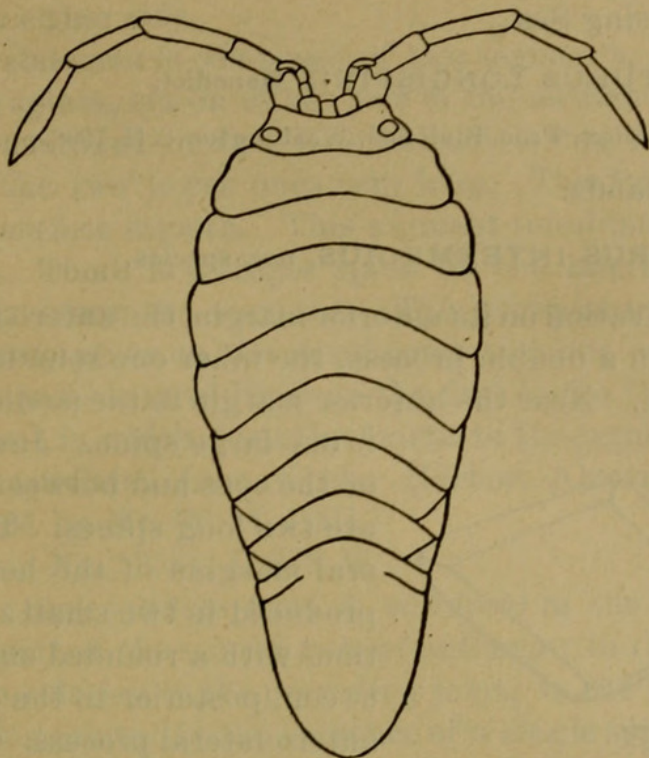
FIG. 26.—EUSYMMERUS ANTENNATUS. X 8.
