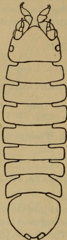
FIG. 32.—JÆROPSIS LOBATA. \times 20 .
