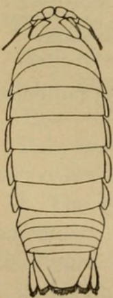
FIG. 5.— ÆGA LECONTII (DANA). × 2.
