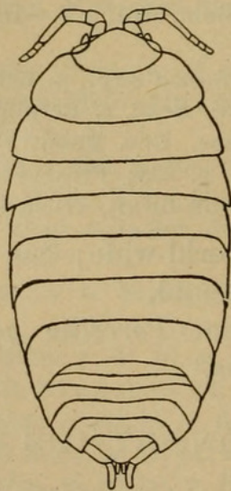
FIG. 34. — ALLONISCUS PERCONVEXUS DANA. × 8.
