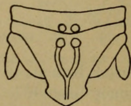
FIG. 12. — SPHÆROMA RHOMBURUM. \times 13\frac{1}{2} . ABDOMEN.
