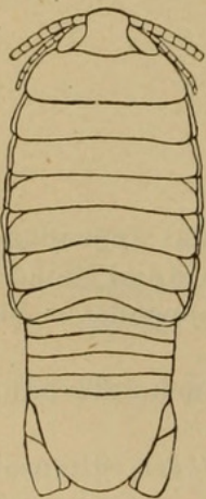
FIG. 7.—ANILOCRA OCCIDENTALIS. \times 4 .
